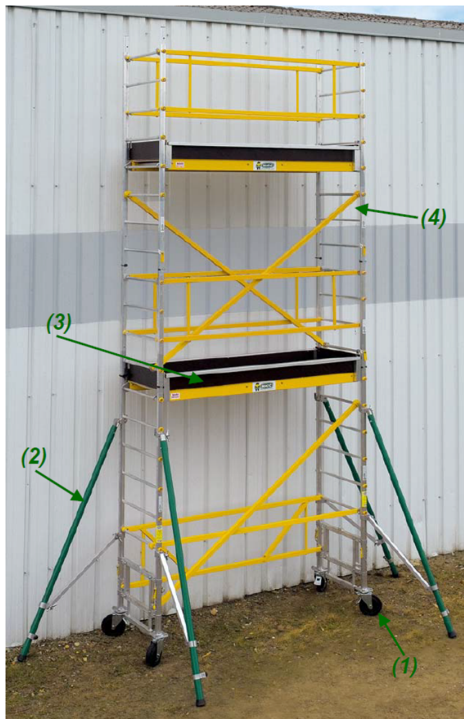
Réglage avec Echafaudage Roulant
